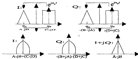
Fig. 8 D_C_M-LO using S_C_M-LO models (spectra).
